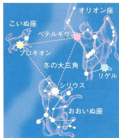
おいぬ座
