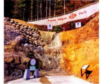
フォッサマグナの断面 (糸魚川市)
